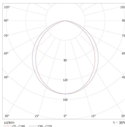
KANLUX S.A. (kat 38897) YALTE D 12 11W WW-B / Krzywa rozsyłu światła (biegunowo)
