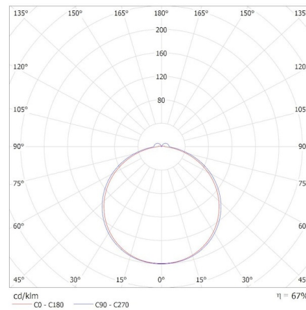
KANLUX S.A. (kat 45819) XERTO EL 20W SE B / Krzywa rozsyłu światła (biegunowo)
