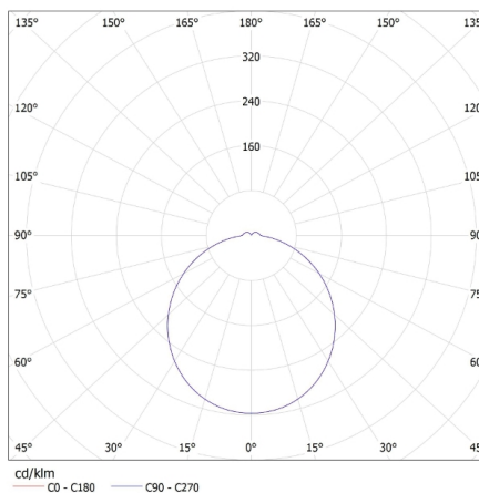
KANLUX S.A. (kat 26981) VARSO LED 18W-NW-O-SE / LDC (Polar)
