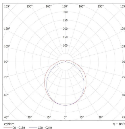
KANLUX S.A. (kat 33169) TP STRONG LED 60W-NW / Krzywa rozsyłu światła (biegunowo)
