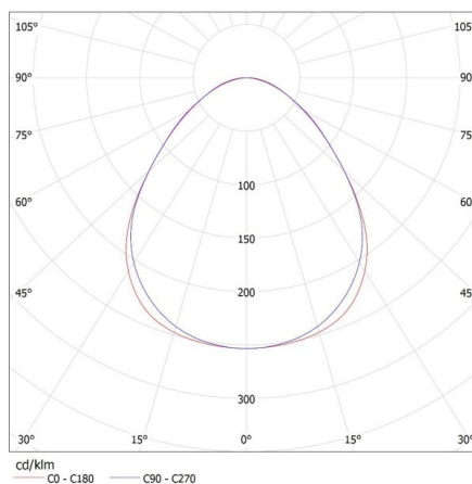
KANLUX S.A. (kat 28451) AL 4LED 120-MPR-SR + GLASSv3 / LDC (Polar)
