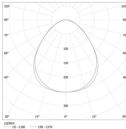
KANLUX S.A. (kat 28451) AL 4LED 120-MPR-SR + GLASSv4 / LDC (Polar)
