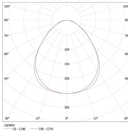
KANLUX S.A. (kat 28452) AL 4LED 150-MPR-W-NT + GLASSv4 / LDC (Polar)
