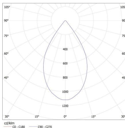
KANLUX S.A. (kat 33136) ATL1 30W-940-S6-W / LDC (Polar)
