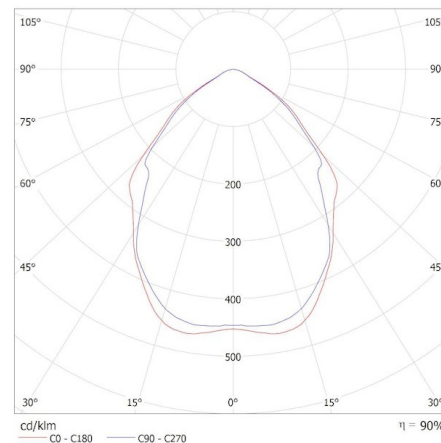
KANLUX S.A. (kat 33138) ATL2 GU10-W + IQ-LED ... 6,5W / Krzywa rozsyłu światła (biegunowo)
