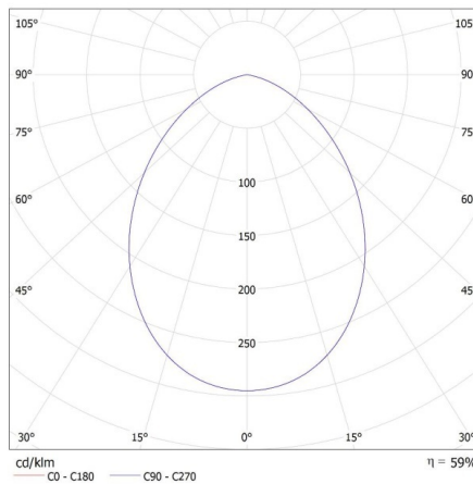
KANLUX S.A. (kat 33362) AQILO IP65 DSO-GR + IQ-LED / LDC (Polar)
