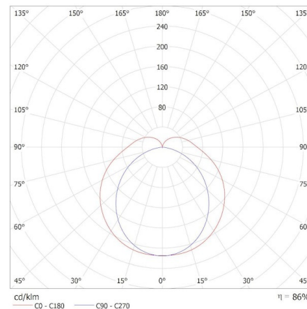
KANLUX S.A. (kat 36659) AKVO IP44 15W-NW-W / Krzywa rozsyłu światła (biegunowo)
