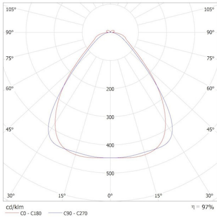
KANLUX S.A. (kat 38391 + 38394) LTL 38W-114-CCT-B 3000K + LENS S 60D / Krzywa rozsyłu światła (biegunowo)
