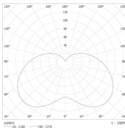
KANLUX S.A. (kat 23438) IDO 6,5W E14-NW / Krzywa rozsyłu światła (biegunowo)
