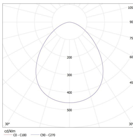
KANLUX S.A. (kat 25781) IVIAN LED 4,5W SN-WW / Krzywa rozsyłu światła (biegunowo)
