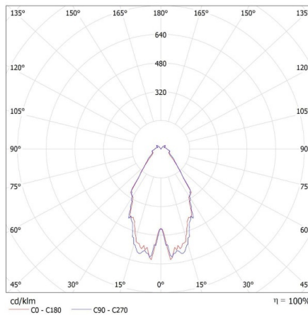
KANLUX S.A. (kat 26047) ST64 A 4W-SW / LDC (Polar)
