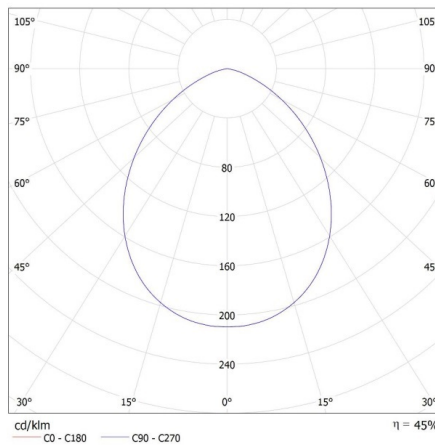
KANLUX S.A. (kat 29232) GOVIK DSO-B/G + IQ-LED ... 6,5W / LDC (Polar)
