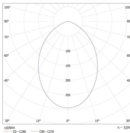
KANLUX S.A. (kat 29232) GOVIK DSO-B/G + IQ-LED ... 6,5WS3 / LDC (Polar)
