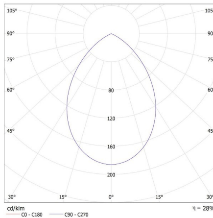
KANLUX S.A. (kat 29236) GOVIK DSO-B + IQ-LED ... 7W / LDC (Polar)
