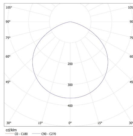
MLEDO (kat 31113) HIBO LED N 150W-NW / LDC (Polar)
