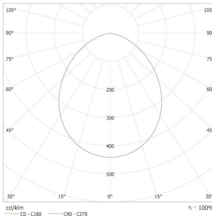
MILED o (kat 31229) GU10 2,7W-CW LED / Krzywa rozsyłu światła (biegunowo)
