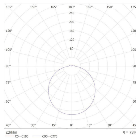
MILED0 (kat 31490) TURA LED 15W-NW-O-B / Krzywa rozsyłu światła (biegunowo)
