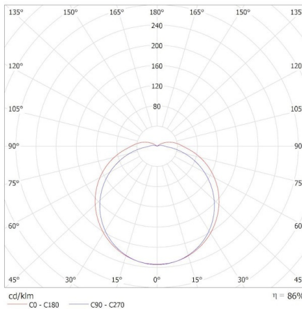
Miledo (kat 31495) TOLU C LED 6W-NW-W / Krzywa rozsyłu światła (biegunowo)
