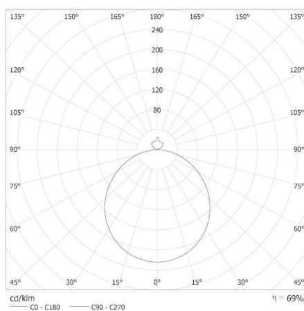
MILED0 (kat 31500) AZPO LED 11,8W-NW-O-W / Krzywa rozsyłu światła (biegunowo)
