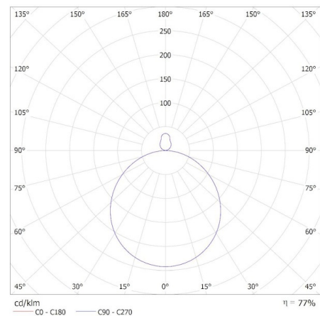
MILEDO (kat 31516) AZPO LED 22WCCT-O-W / Krzywa rozsyłu światła (biegunowo)
