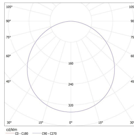
KANLUX S.A. (kat 33532) CARSA V2LED 12W-NW-B / LDC (Polar)
