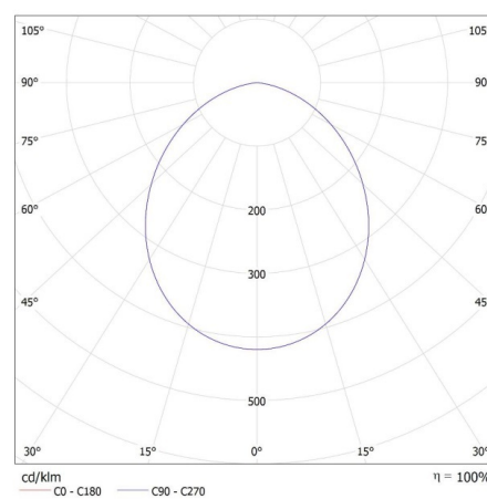
KANLUX S.A. (kat 34965) TOMiv2 2,9W GU10-WW / LDC (Polar)
