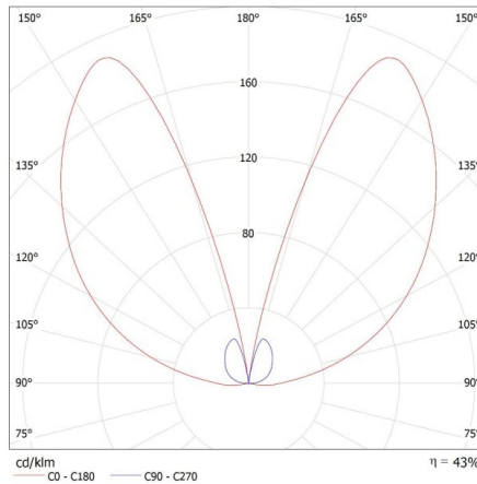
KANLUX S.A. (kat 36550) PEVO 80 GR + ESG LED 9W / LDC (Polar)
