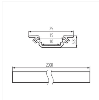
PROFILO E 2m
