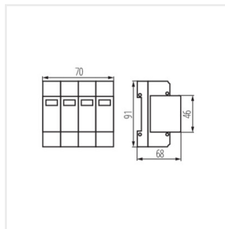
KSD-T1T2 275/240 3P+N
