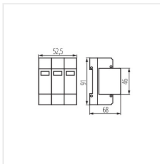
KSD-T1+T2 275/180 3P
