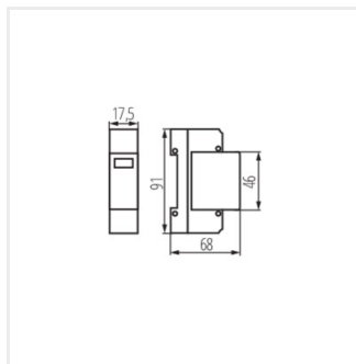
KSD-T1+T2 275/60 1P
