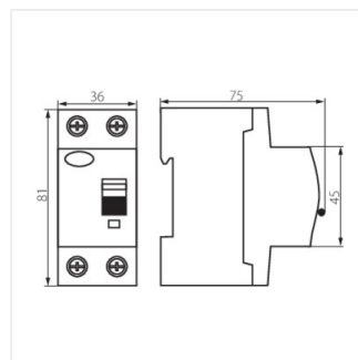
KRD6-2/16/10-A
