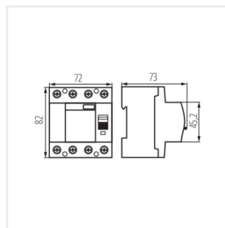
KRD10-4/63/30-A
