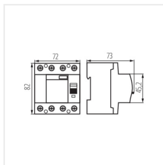
KRD10-4/40/30-AC
