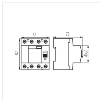
KRD10-4/63/30-AC
