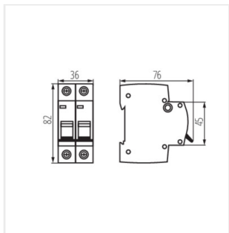
KMB10-B20/2
