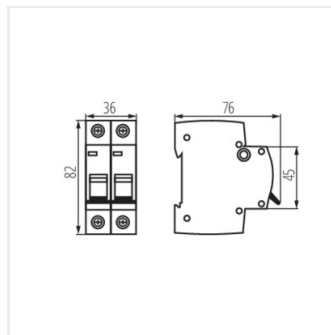
KMB10-B10/2
