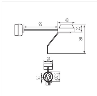
BR-GZ10
