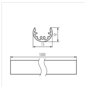
PROFILO A
