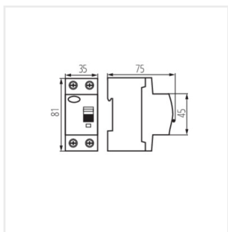
KRD6-2/16/10-A
