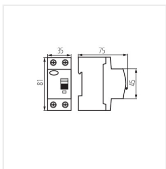
KRD6-2/16/10
