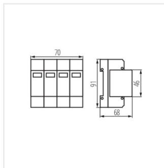
KSD-T2 275/160 3P+N
