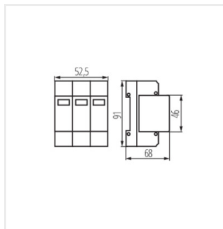
KSD-T2 275/120 3P
