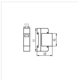
KSD-T2 275/40 1P
