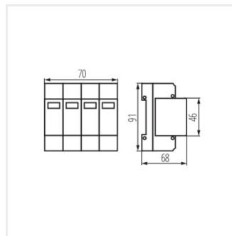
KSD-T1T2 275/240 3P+N
