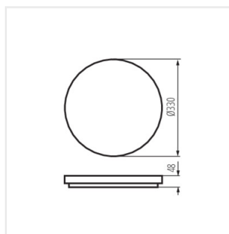
VARSO 22-30W-CCT-O
