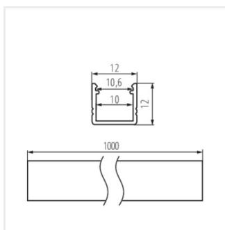
PROFILO F
