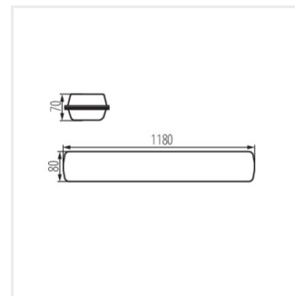
FTD1200 37W-840-ASY
