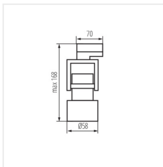
ATL5 GU10-B
