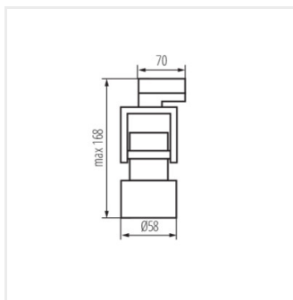
ATL5 GU10-W
