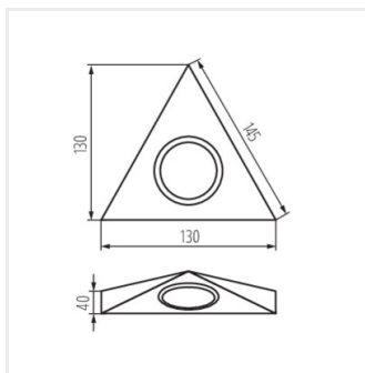
ZEPO LFD-T02
