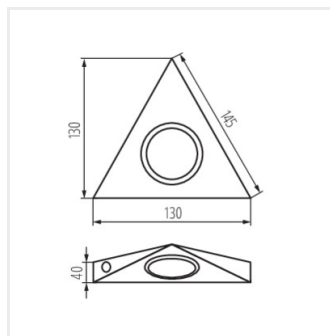
ZEPO LFD-T02/S-C/M
