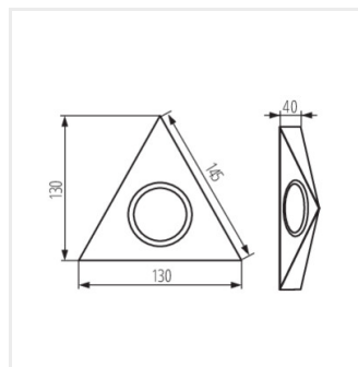
ZEPO LFD-T02-W
