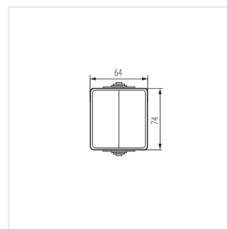
TEKNO IP65GR 2G1W
