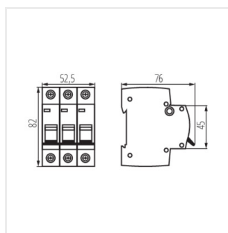
KMB10-C32/3
