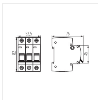
KMB10-C25/3
