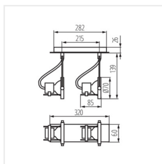
SONDA EL-2J
