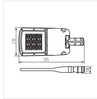
PRO-S S 35W-ZH NW
