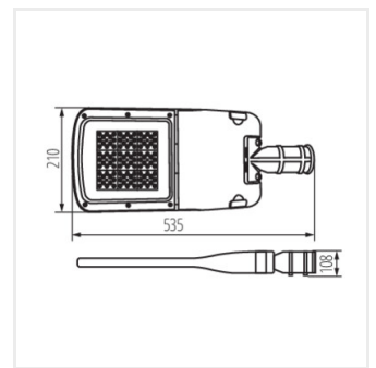
PRO-S S 65W-ZH NW
