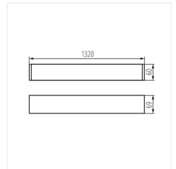
AL 4LED 1X120-B SE
