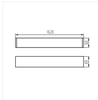
AL 4LED 1X150-B SE
