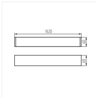
AL 4LED 1X150-B-NT SE
