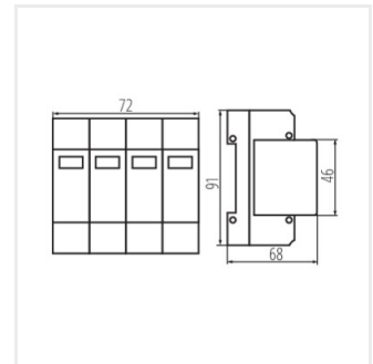
KSPD-TT 275/160 3P+N
