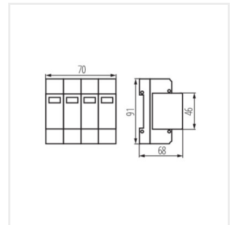
KSD-T1T2 275/240 3P+N
