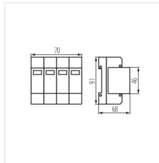
KSD-T2 275/160 3P+N
