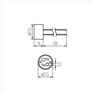
HLDR-GZ10
