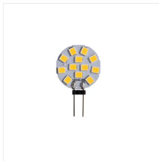
LED12 G4-NW
