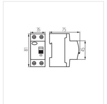
KRD6-2/16/10-A
