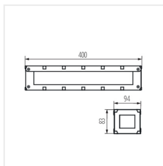
KP-DB-I-MF CON-V-M
